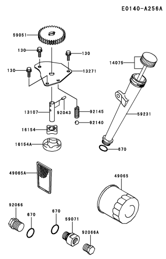
B-06 LUBRICATION-EQUIPMENT
